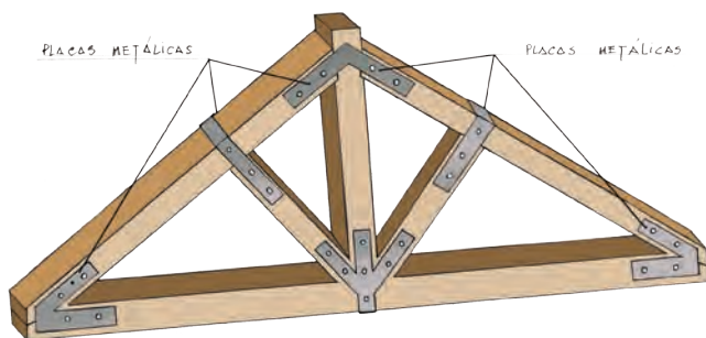
REFORZAMIENTO DE ESTRUCTURA DE MADERA
