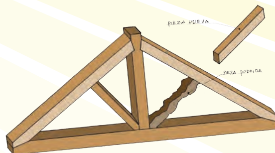
SUSTITUCIÓN DE ELEMENTO COMPROMETIDO
