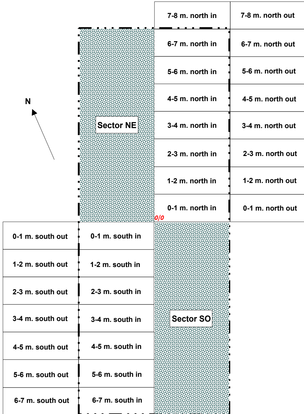
FIGURA 3.5: Representación esquemática de las unidades excavadas en la Estructura 1
