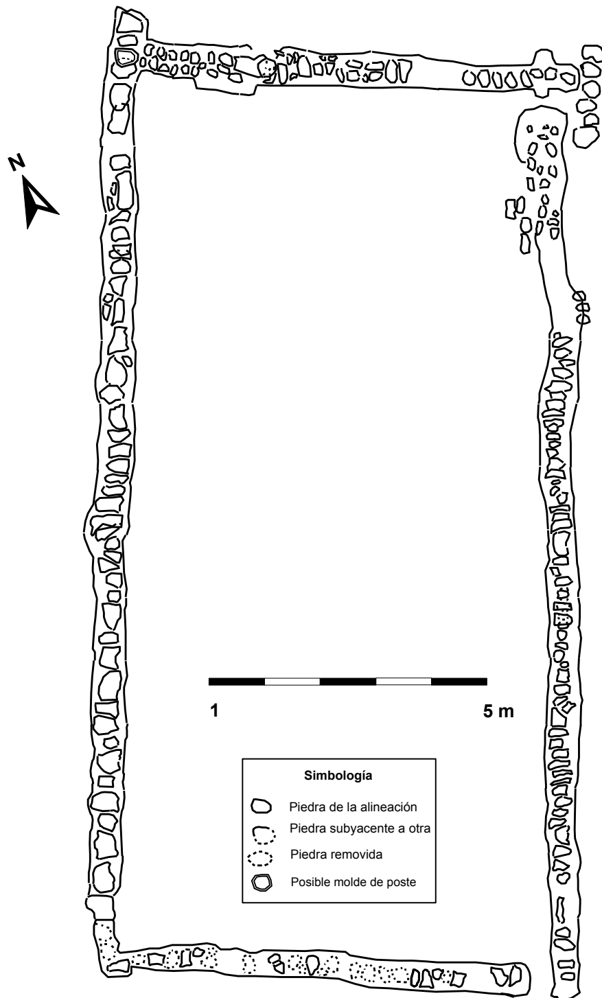
Figura 3.2.: Alineación de Piedras de la Estructura 1 sitio OMJPLP-15, Puerto López Viejo
