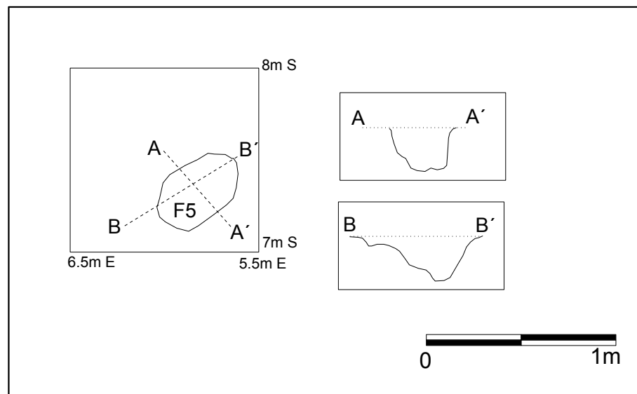
Figura 5.2: Planta y cortes del rasgo 5
