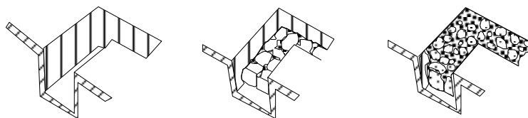
Figura 5.1: Construcción de los Cimientos para la técnica de Tapial
